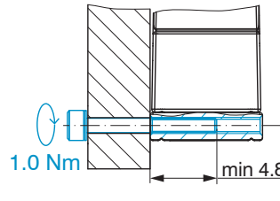
Washer A3,2; ISO 7089 - A2 M3; ISO 4762-A2
