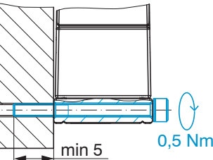
Washer A2,2; ISO 7089 - A2 M2 x 25; ISO 4762-A2
