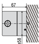
Ausgang P200-HTL/TTL
