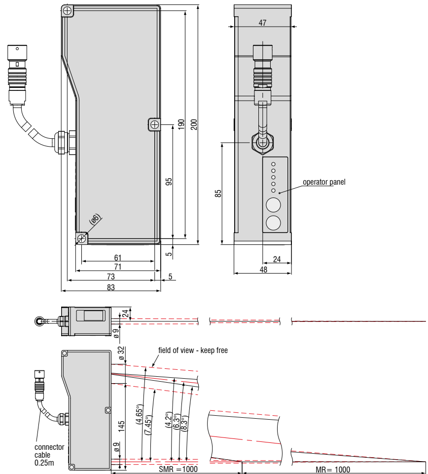
optoNCDT 1710-1000
