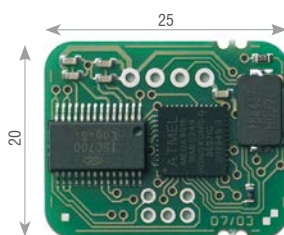
ISC7001 Électronique de platine miniature
