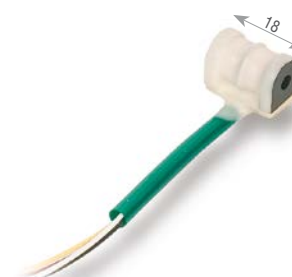
DTA-1D-20-DDV.02 Capteur de déplacements LVDT avec bobine immergée
