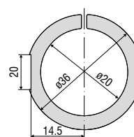
MA 2406-20 for sensors IFS2406-2,5 IFS2406/90-2,5
