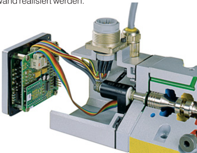
Induktive Wegsensoren (LVDT-Prinzip) in Hydraulikventilen der Fa. MOOG
